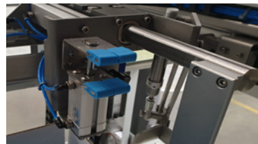
Pinças mecânicas e colheres
